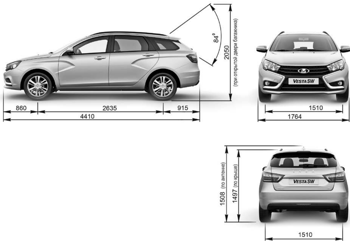
Рис. 4. Габаритные (справочные) размеры автомобиля Vesta SW (в варианном исполнении)
